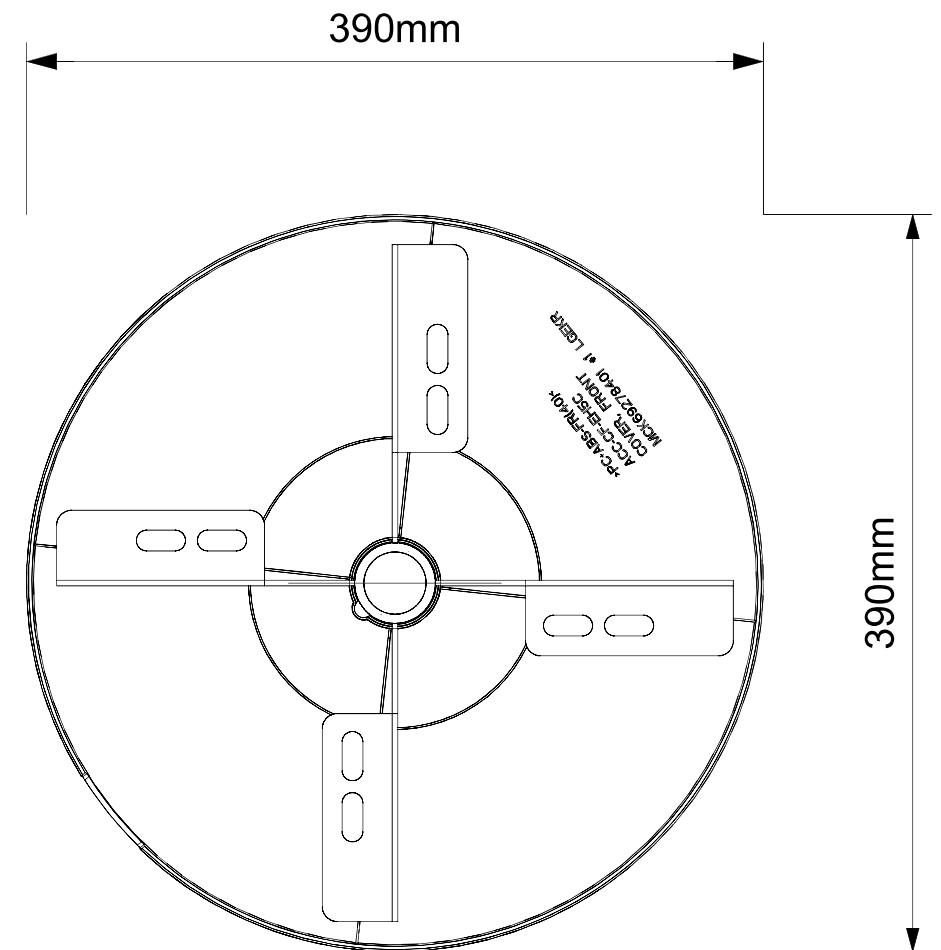
3 Ansicht Oben Maßstab: 1:4
