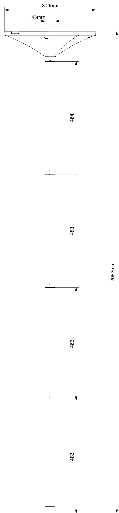
1 Ansicht Vorne Maßstab: 1:10
