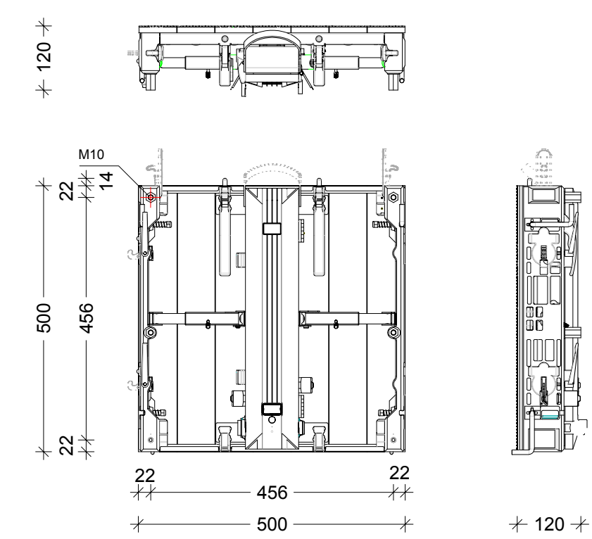
Detailansicht
