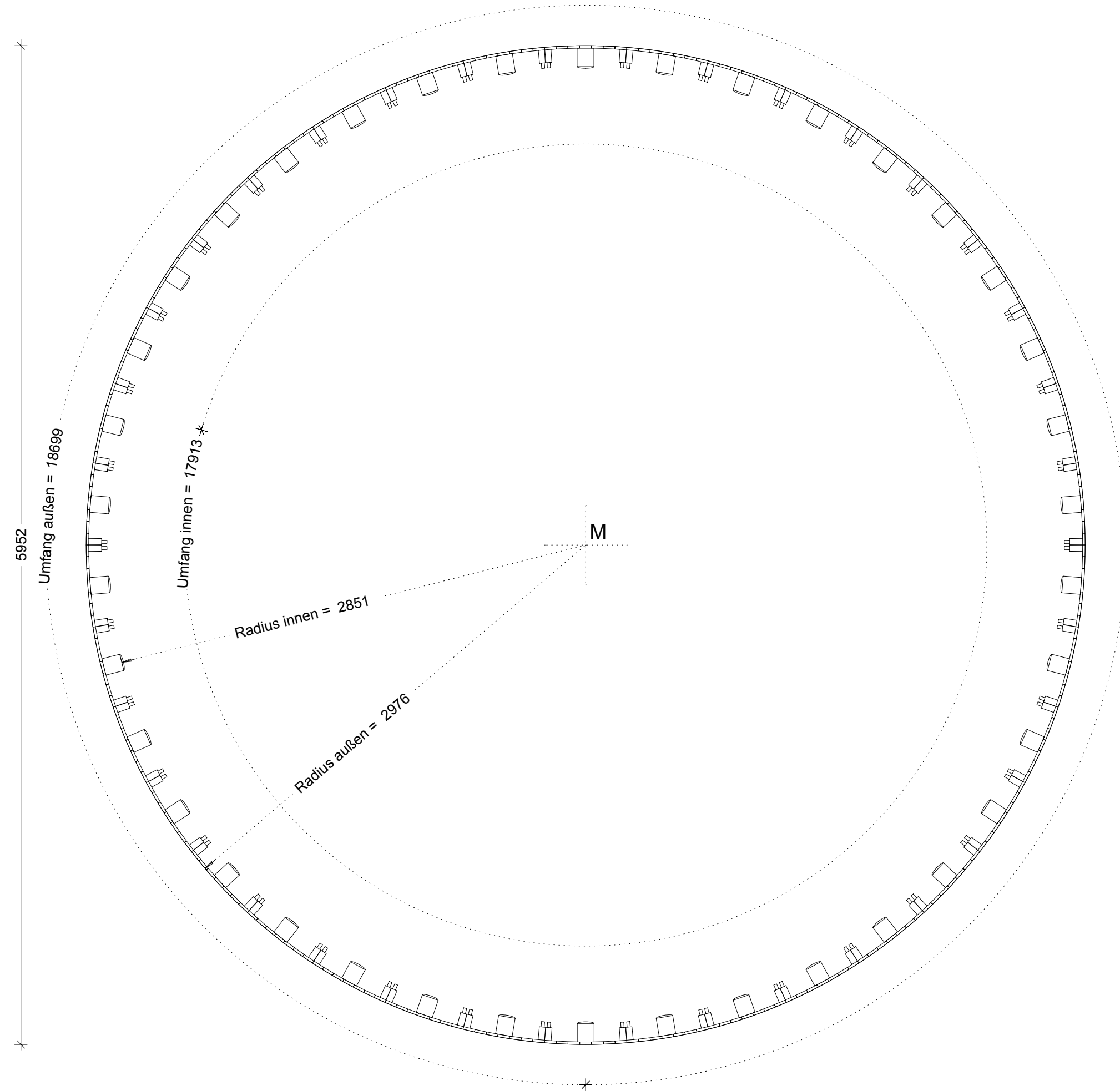
Draufsicht
